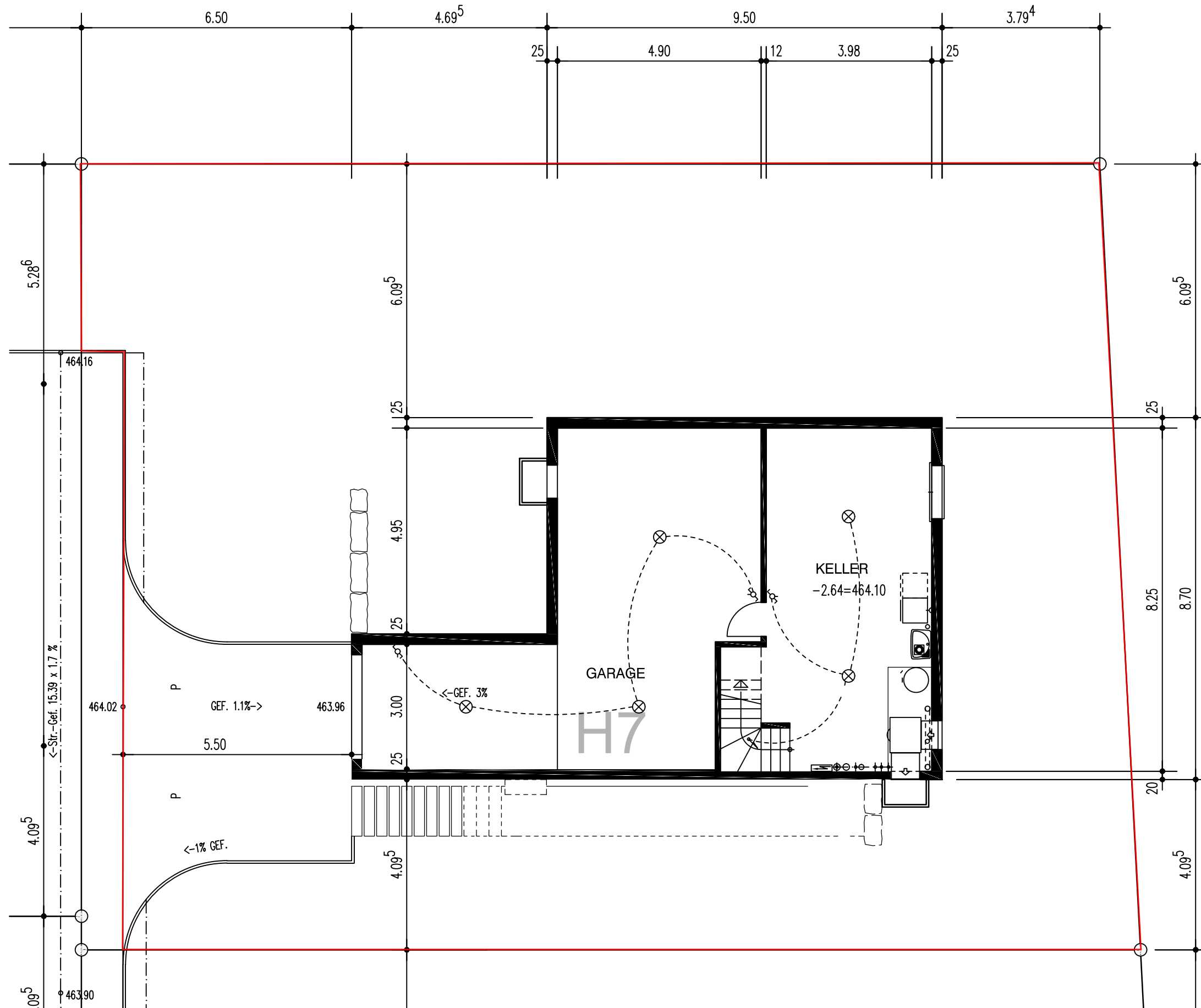
UNTERGESCHOSS H7 1:100
