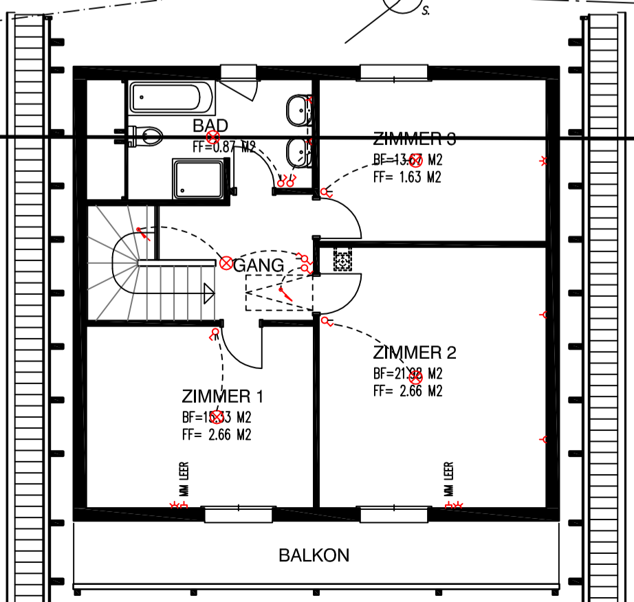
NORM OBERGESCHOSS FÜR 5 HÄUSER
