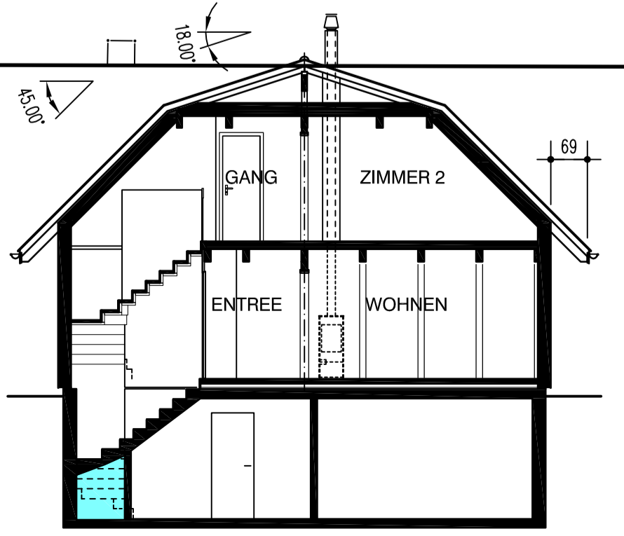
NORM SCHNITT FÜR 5 HÄUSER
