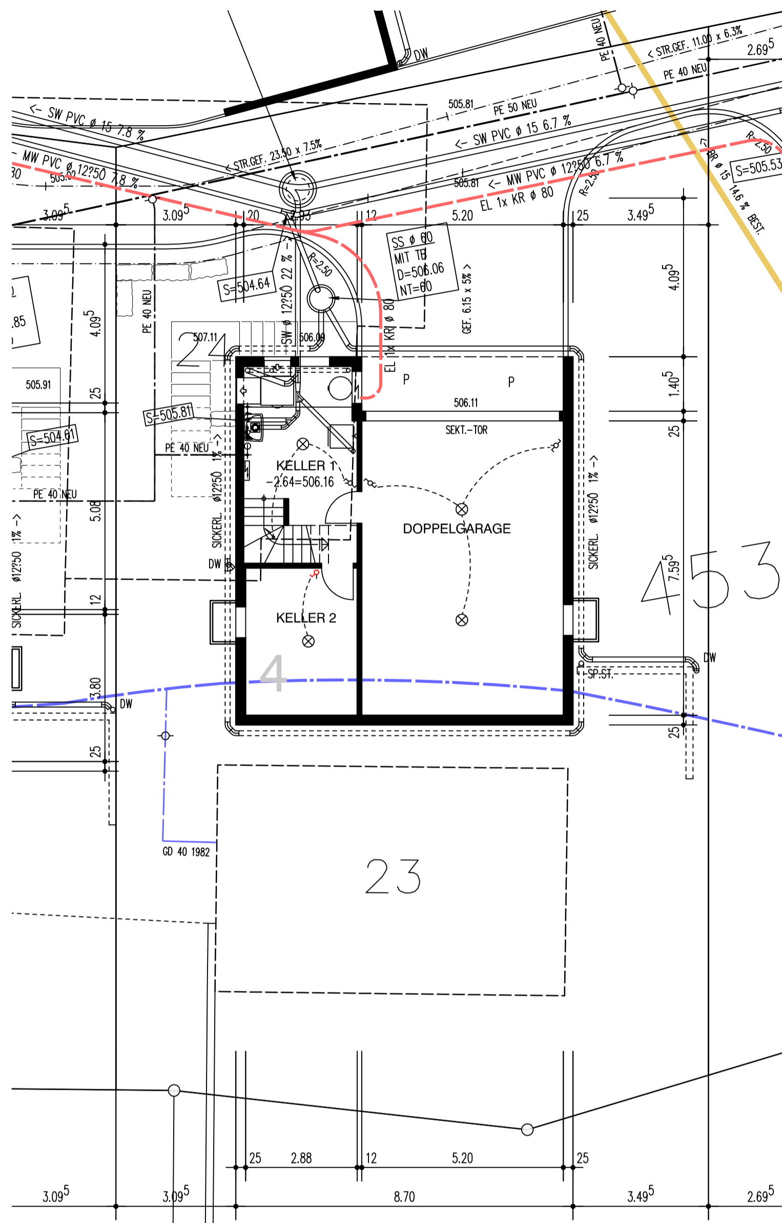
UNTERGESCHOSS
