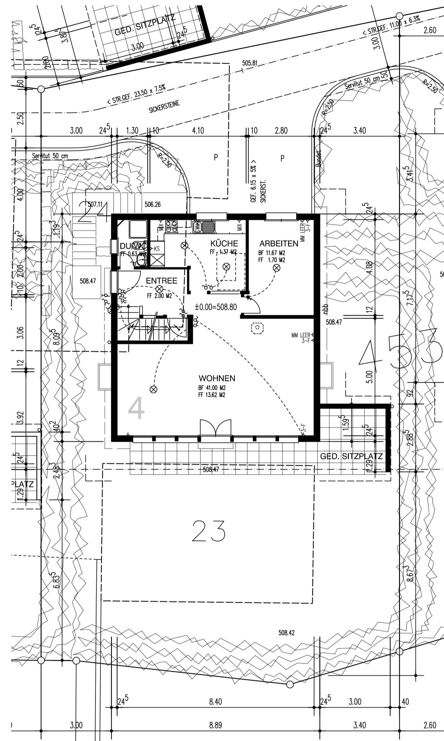
ERDGESCHOSS
