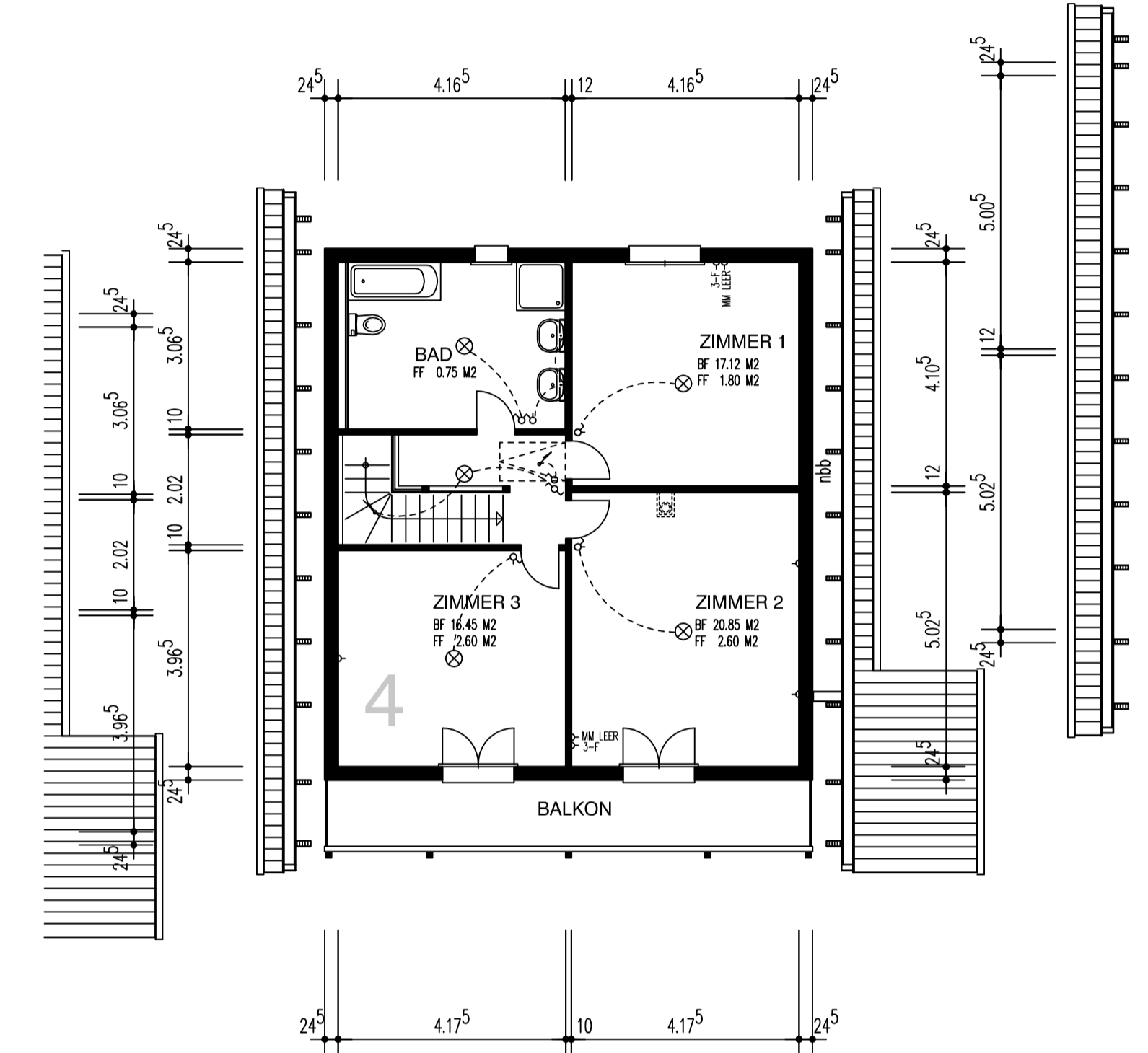
OBERGECHOSS
