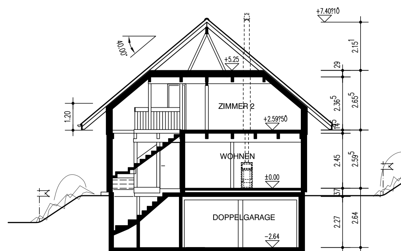
QUERSCHNITT
