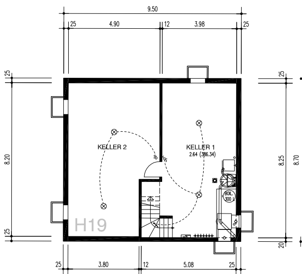
UNTERGESCHOSS
