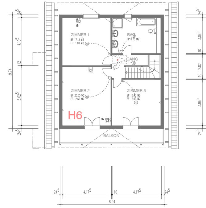
OBERGESCHOSS
