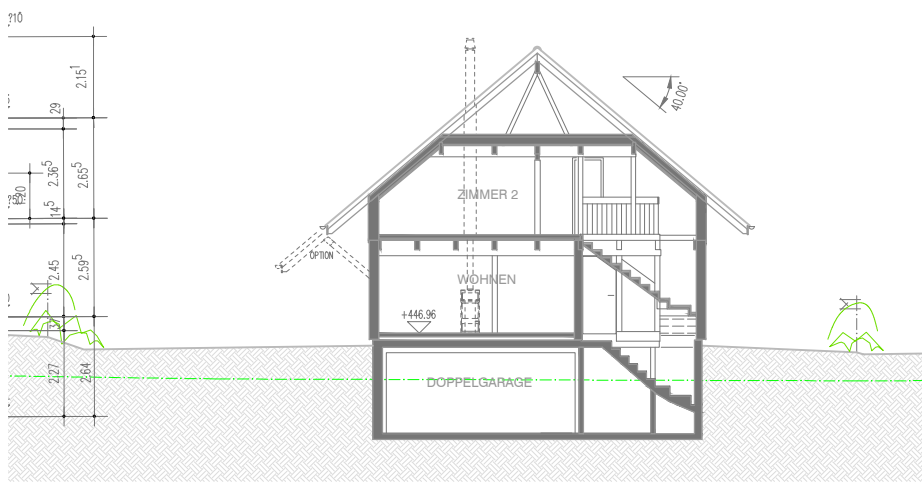
QUERSCHNITT
