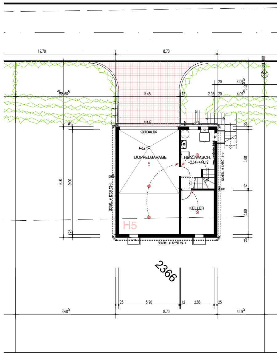
UNTERGESCHOSS
