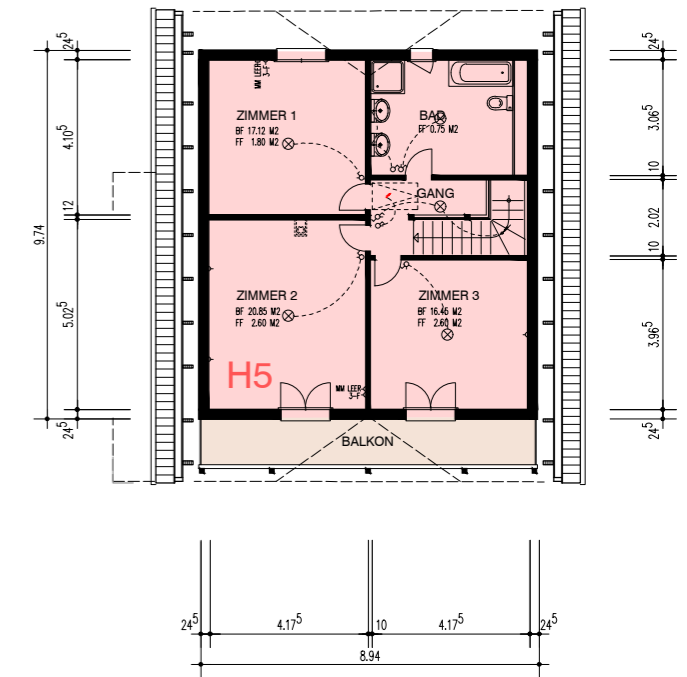
OBERGESCHOSS
