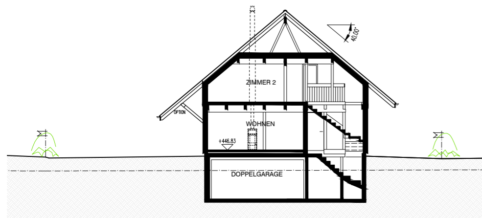
QUERSCHNITT
