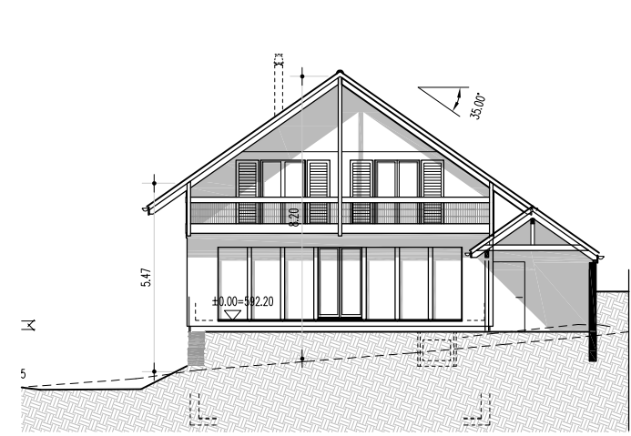
M4 SÜDWESTFASADE
