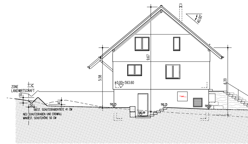
M5 NORDOSTFASADE
