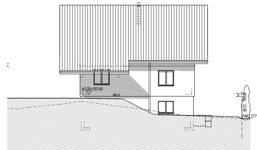
M5 SÜDOSTFASADE
