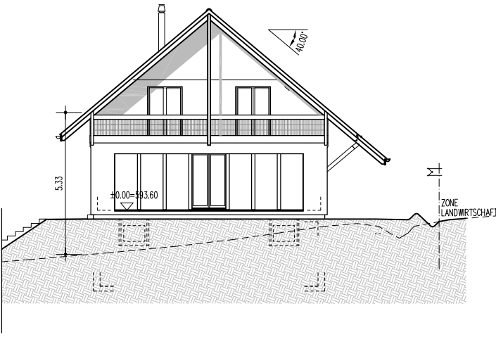
M5 SÜDWESTFASADE
