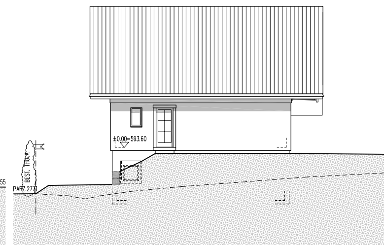
M5 NORDWESTFASADE
