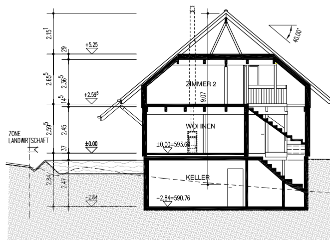
M5 SCHNITT
