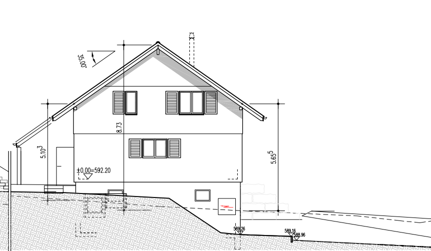
M4 NORDOSTFASADE
