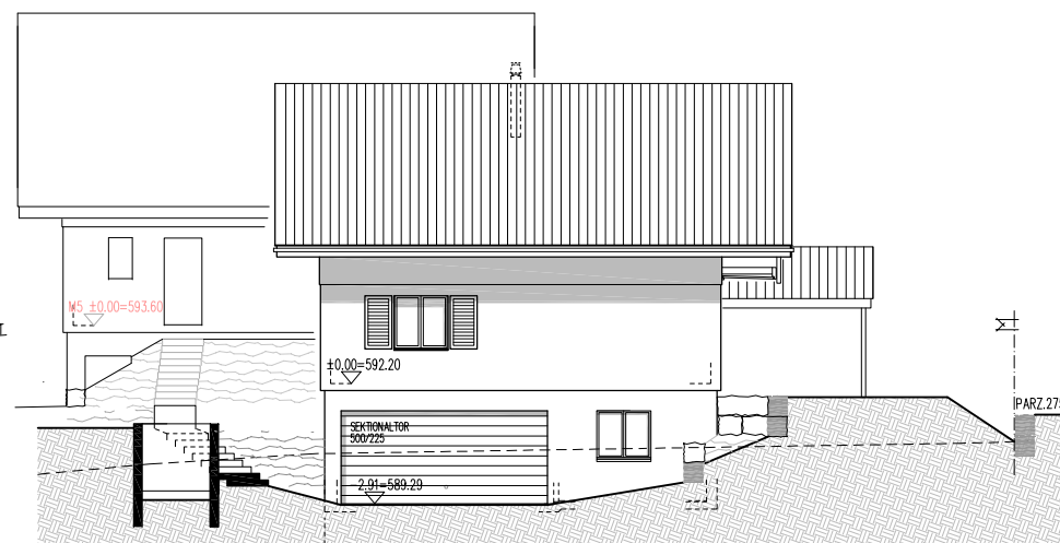
M4 NORDWESTFASADE
