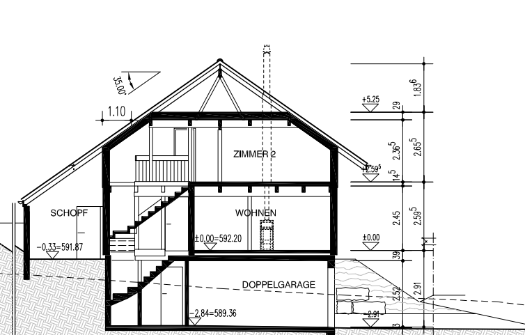
M4 SCHNITT
