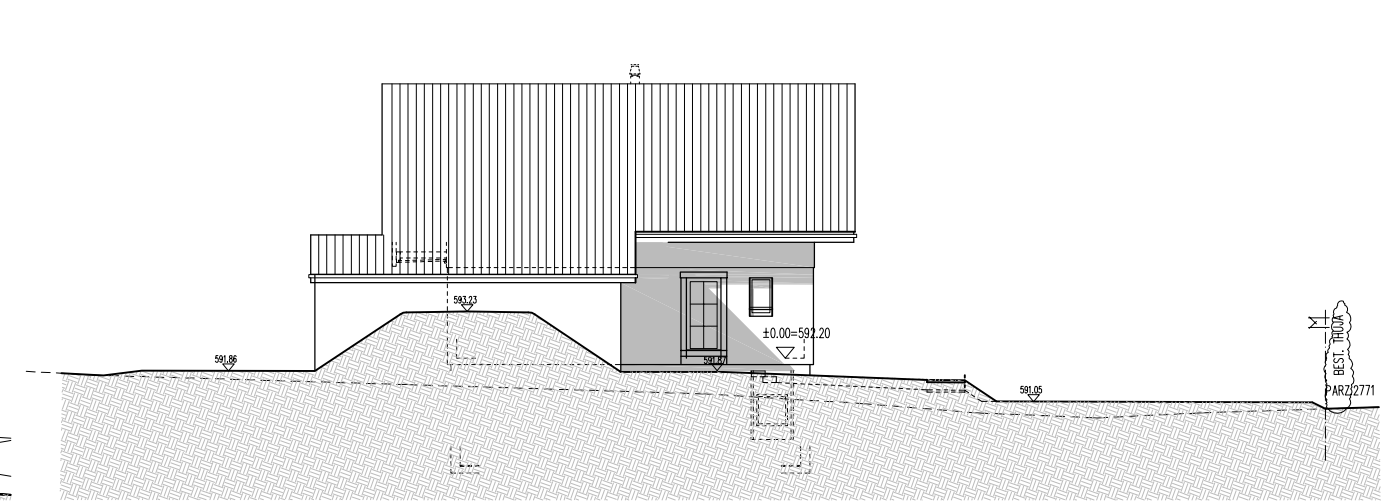
M4 SÜDOSTFASADE
