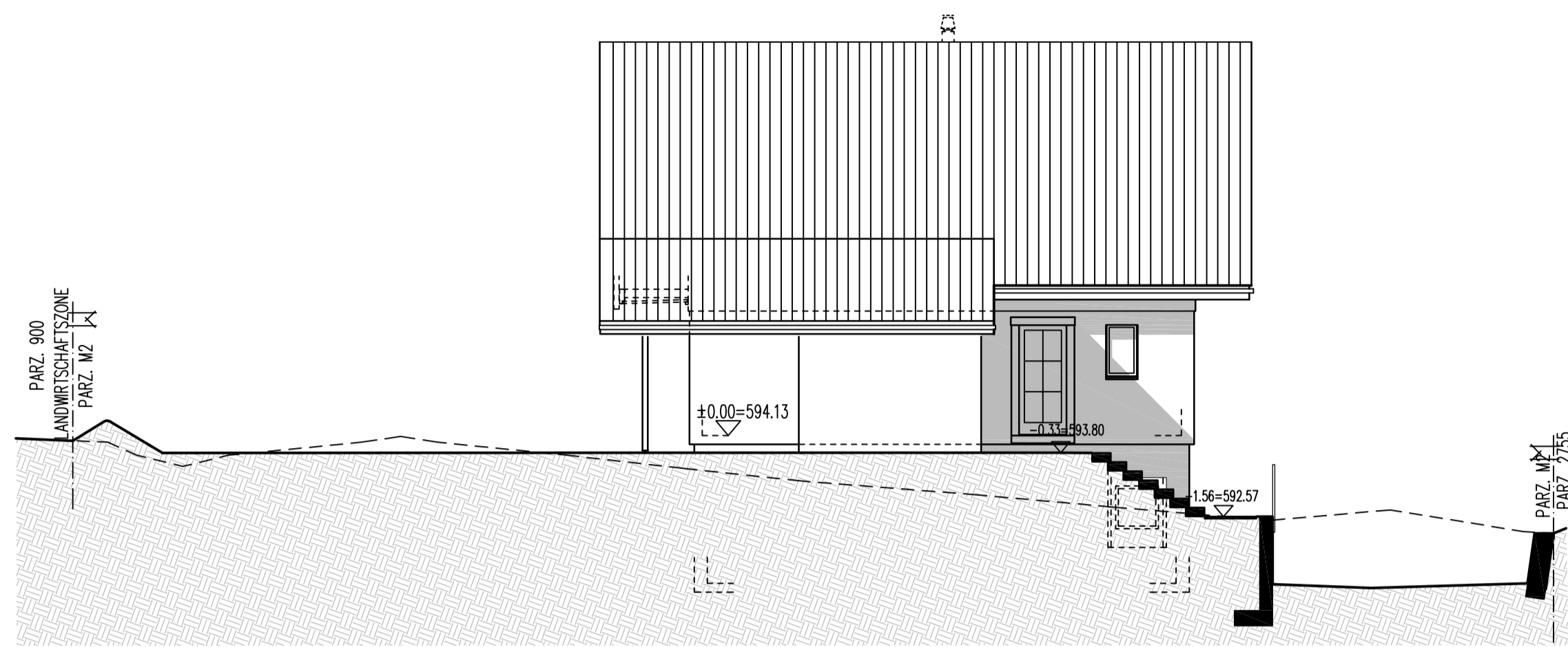
M2 OSTFASSADE
