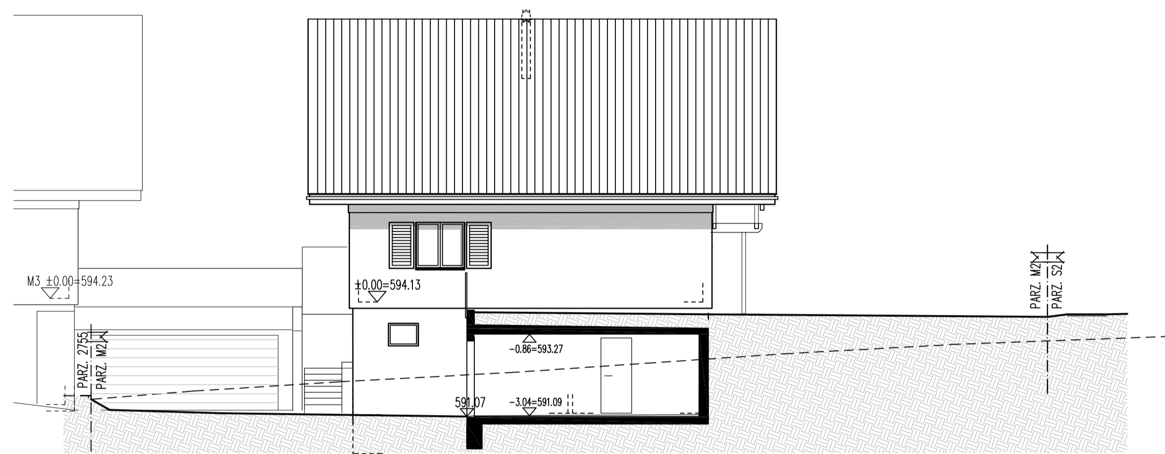
M2 WESTFASSADE
