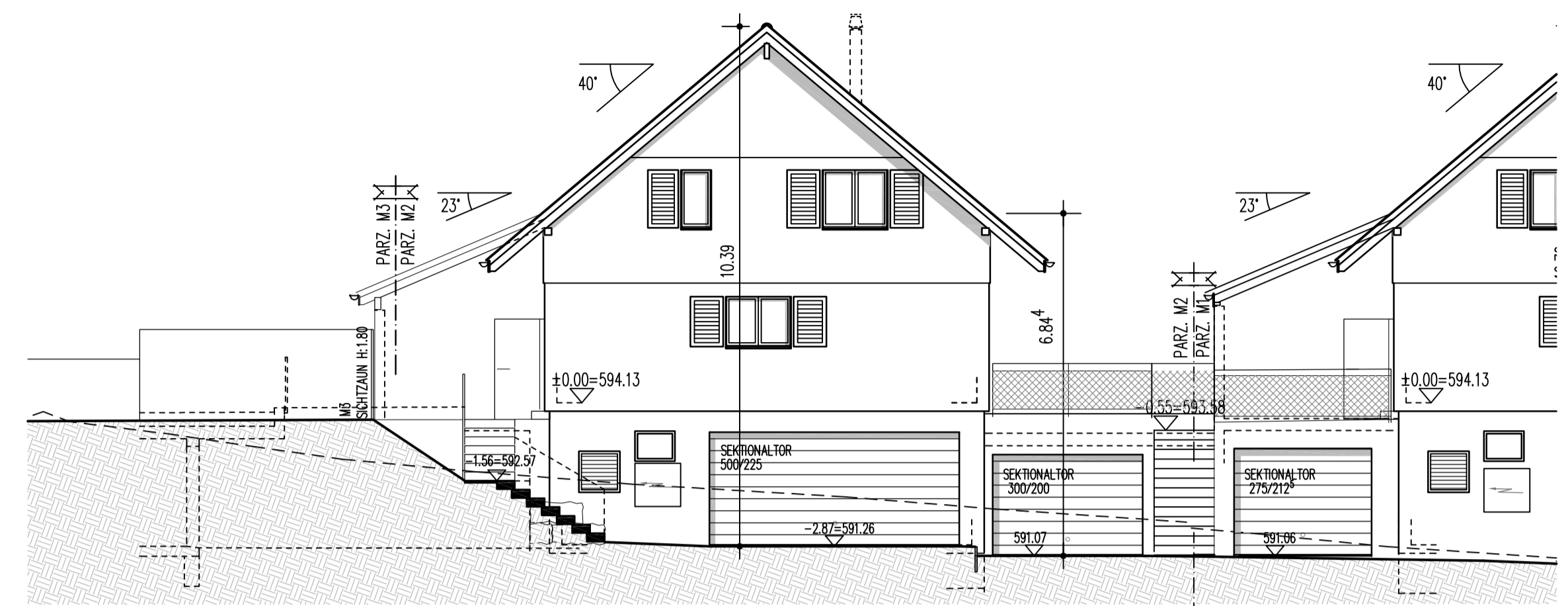
M2 NORDFASSADE
