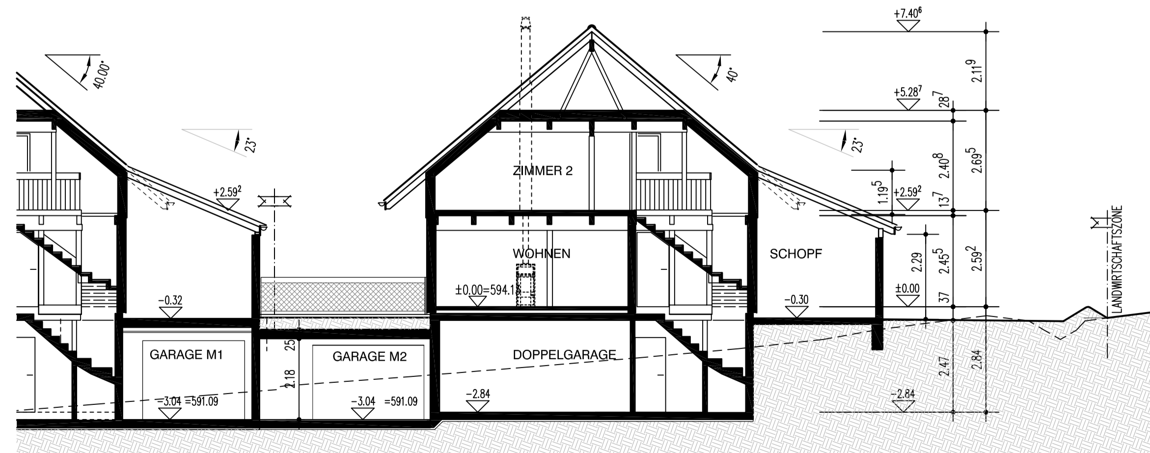
M2 SCHNITT
