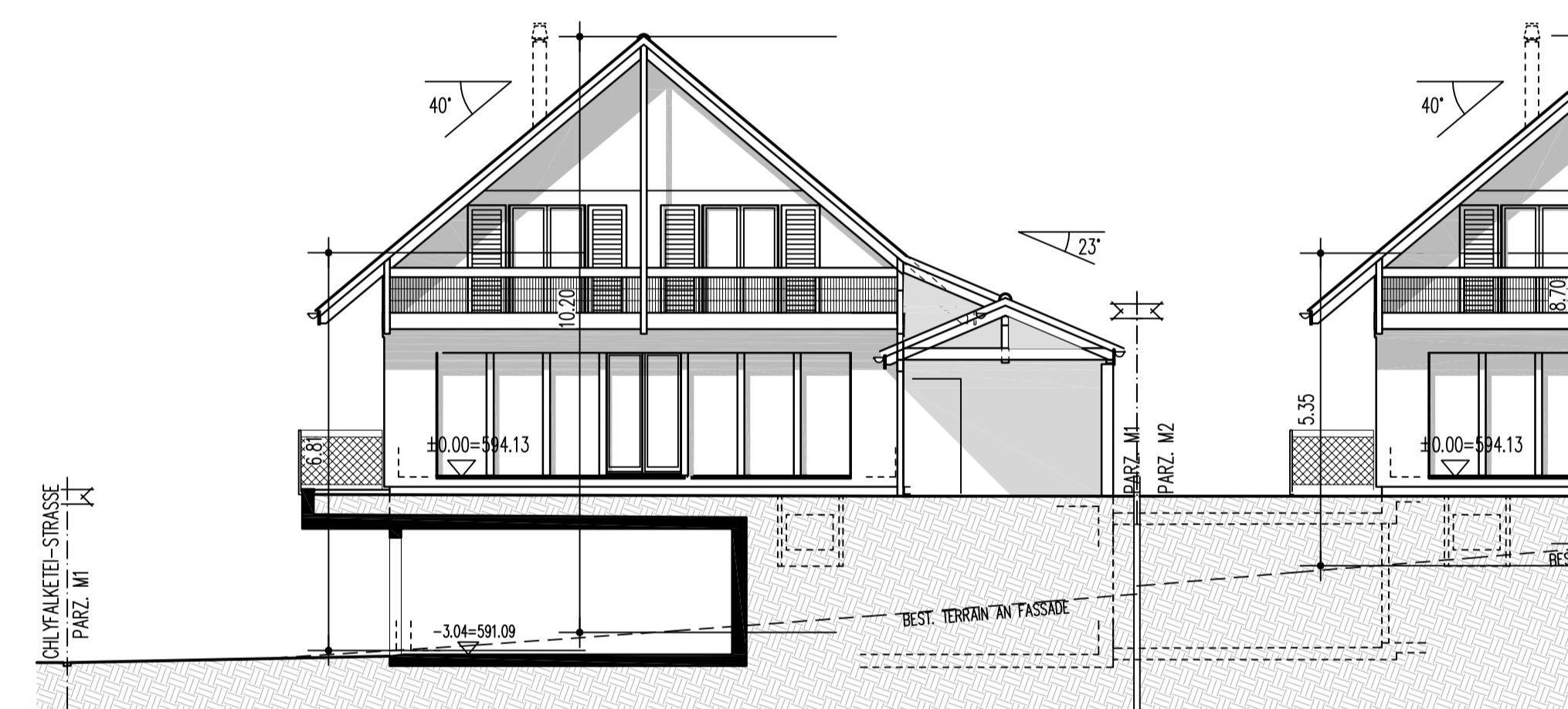
M1 SÜDFASSADE
