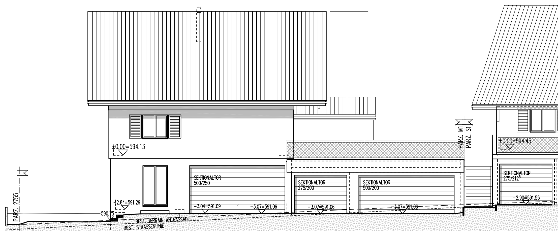
M1 WESTFASSADE
