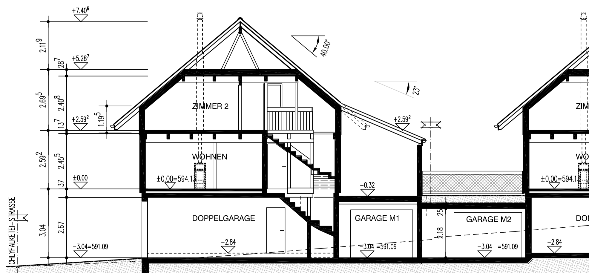
M1 SCHNITT
